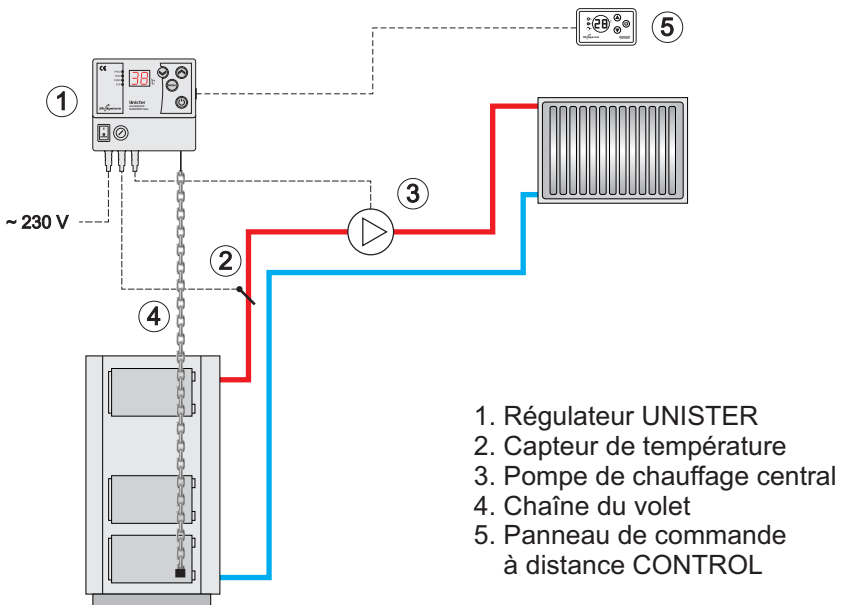
Fig.1 Raccordement du régulateur au système de chauffage central
