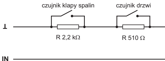
Rys. 4 Schemat połączenia czujników klapy spalin i drzwi. Dokładny opis w punkcie 34 instrukcji.
