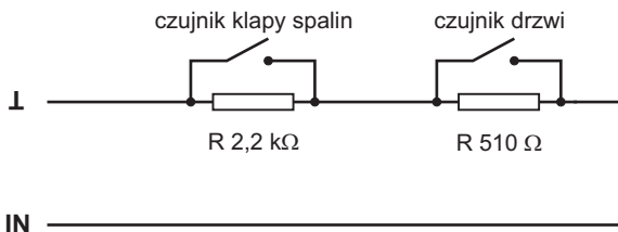
Rys. 6 Schematy obwodów czujników
