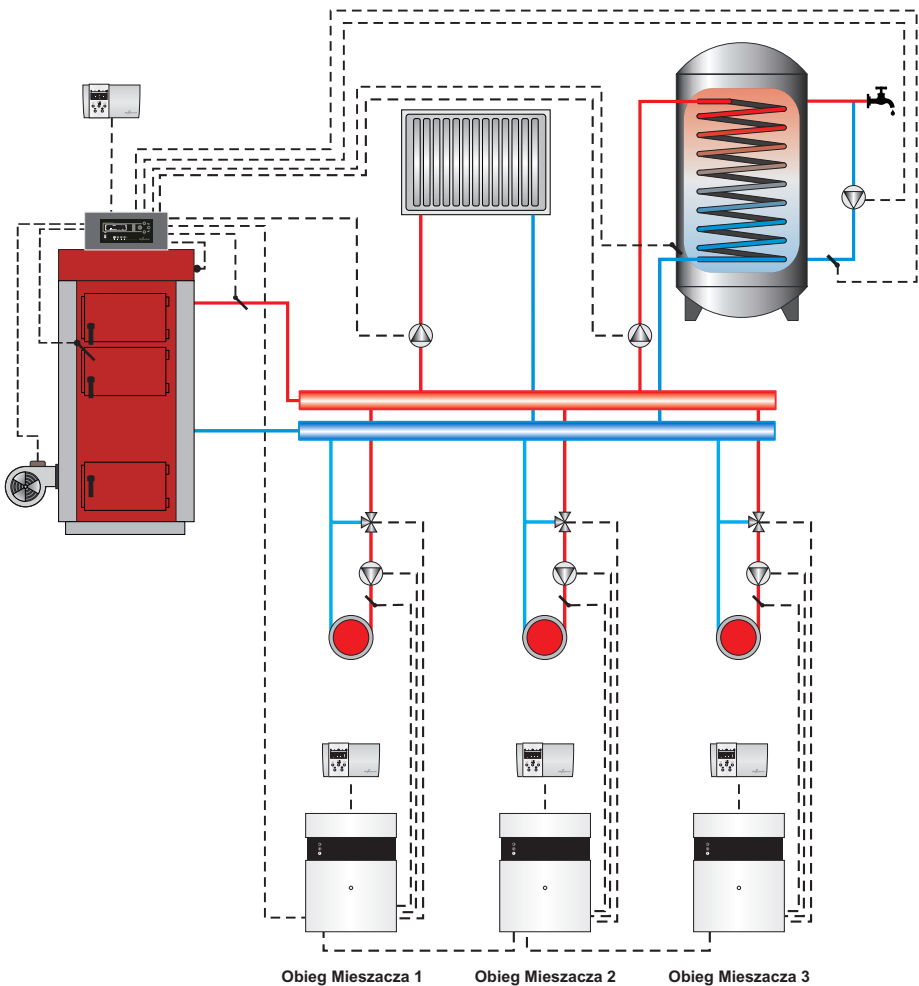
Rys. 5 Przykładowy schemat instalacji z podłączonymi trzema modułami rozszerzającymi DKMZ: Obiegu Mieszacza 1 , Obiegu Mieszacza 2 i Obiegu Mieszacza 3 .
