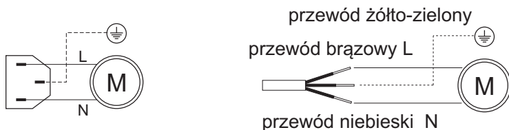
Rys. 3 Schematy podłączenia przewodu zasilającego do wentylatora i pomp (w zależności od wersji regulatora)
