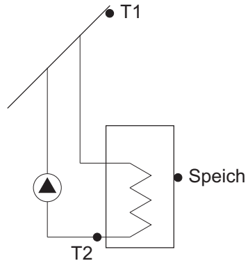
Abb. 5 Schema der Sensorinstallation - Option T2.
