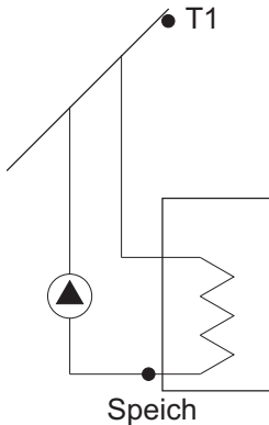
Abb. 4 Schema der Sensormontage - Option Speich.
