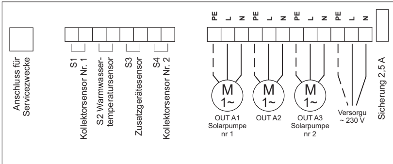
Abb. 1 Elektrischer Schaltplan zum Anschließen der Stromkabel
