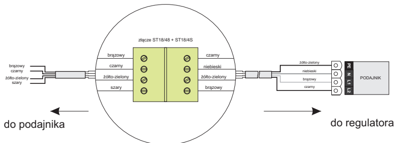
Rys. 6 Schemat podłączenia przewodu do podajnika
