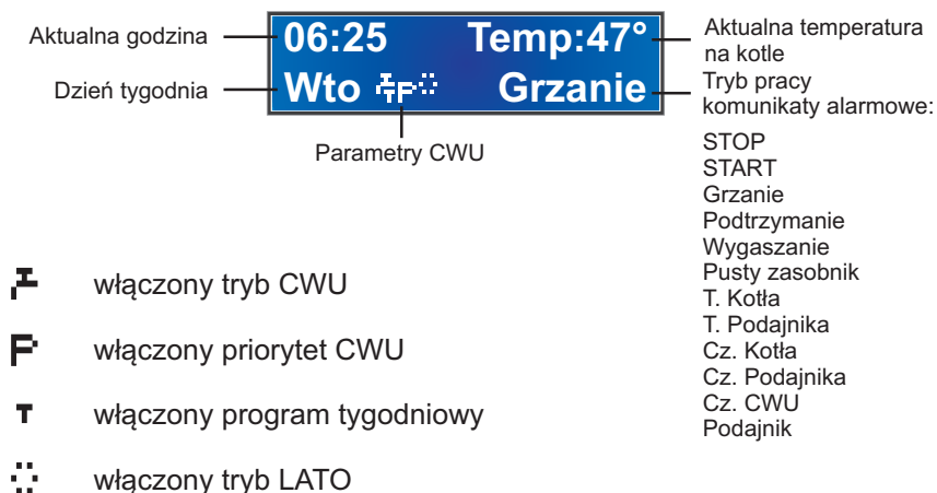
Rys. 2 Opis ekranu roboczego
