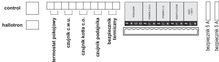
Rys. 3 Schemat elektryczny podłączenia czujników i przewodów zasilających
