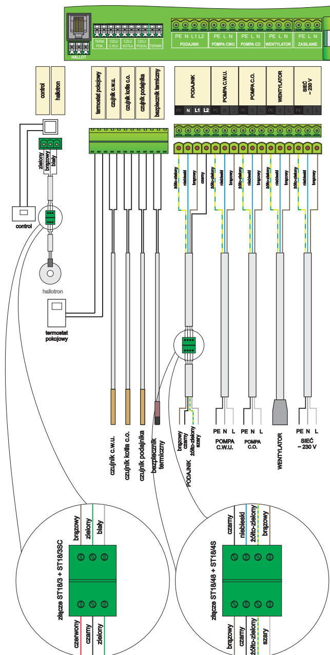
Rys. 7 Schemat elektryczny złącz wyjściowych i kabli przyłączeniowych
