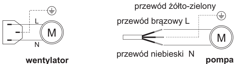
Rys. 5 Schematy podłączenia przewodu zasilającego do wentylatora i pompy
